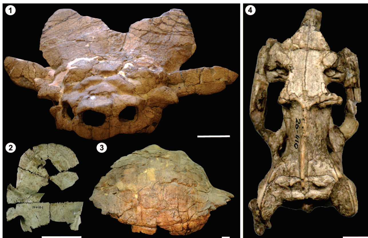
Figura 6. Reptiles no arcosaurios continentales icónicos del MLP. 1, Neotipo de Niolamia argentina (MLP-26-40), cráneo en vista anterolateral; 2, Holotipo de Acanthochelys cosquinensis (MLP-77-V-12-1), plastrón en vista dorsal; 3, Holotipo de Chelonoidis australis (MLP-26-400); 4, Holotipo de Dinilyisia patagonica (MLP 26-410). Escala= 5 cm (1); 10 cm (2, 3); 1 cm (4).
