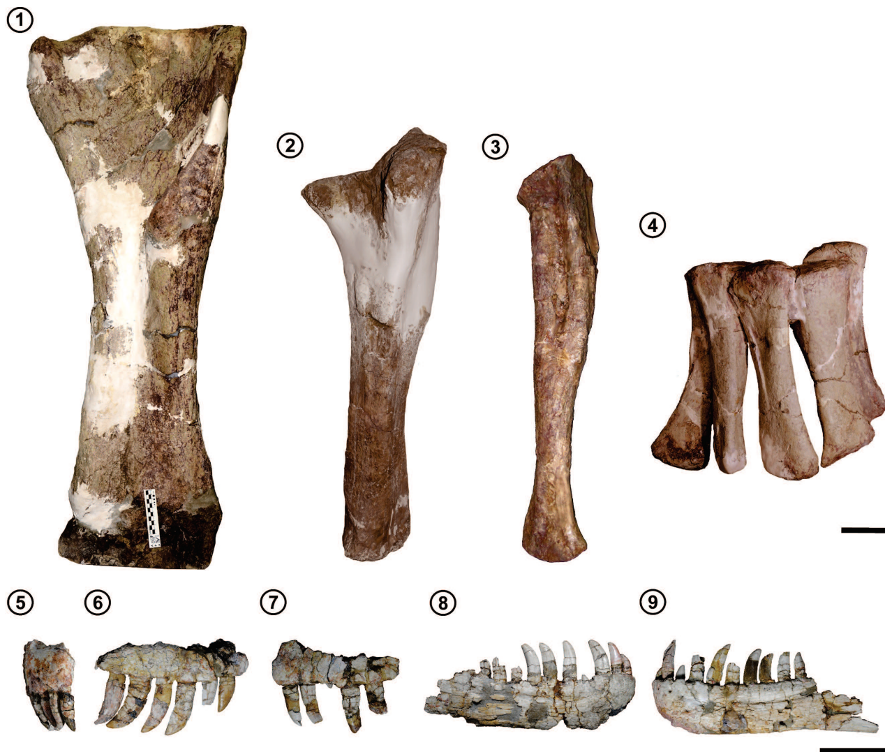
Figura 3. Algunos materiales holotípicos de dinosaurios del MLP. 1–4, Argyroosaurus superbus (MLP 77-V-29-1). 1, húmero izquierdo en vista anterior; 2, ulna izquierda en vista anterolateral; 3, radio izquierdo en vista posterior; 4, metacarpo izquierdo en vista anterior. 5–9, Genyodectes serus (MLP 26-29); 5, premaxila izquierda en vista lateral; 6, maxila derecha en vista lateral; 7, maxila izquierda en vista lateral; 8, dentario derecho en vista lateral; 9, dentario izquierdo en vista lateral. Escala= 10 cm.
